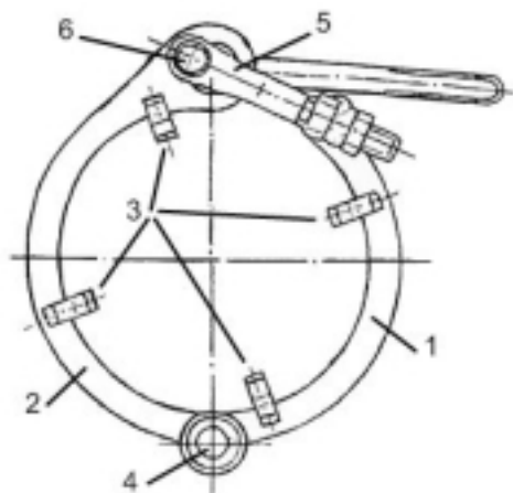
6 и 5 - эксцентрик, 3 - центрирующие надставки (опоры), 4 - ось, 5 - тяга с перекладиной
